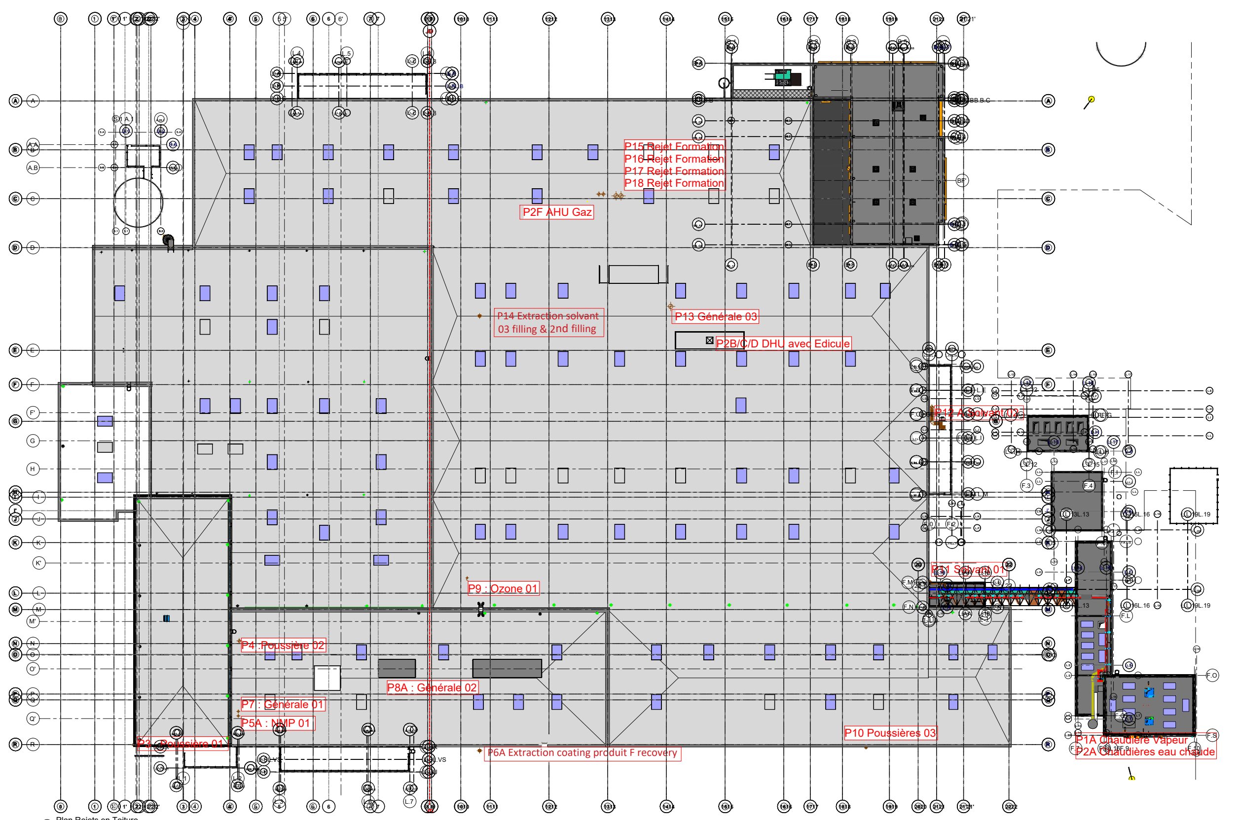
1 Plan Rejets en Toiture 1 : 200
